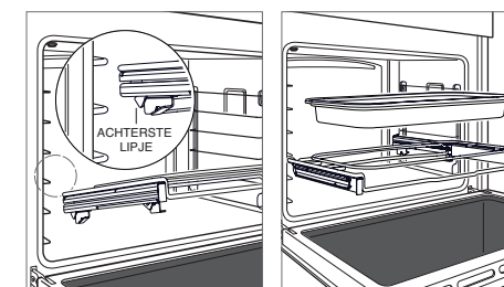
Installeer multifunctioneel rek
