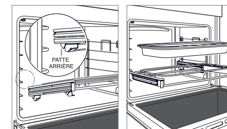
Installez la grille multifonctions
