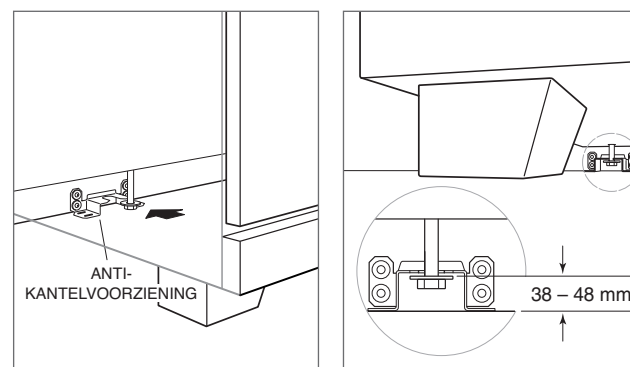
Locatie anti-kantelvoorziening
