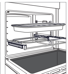
Multifunktionspfanne darauf stellen
