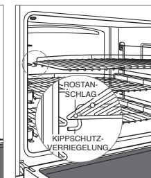
Kippschutzverriegelung des Backofenrostes
